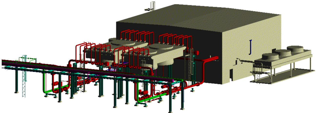
Bild: NW Ansicht Hochdruckverdichterhalle mit Gaskühler und Rohrbrücke.
